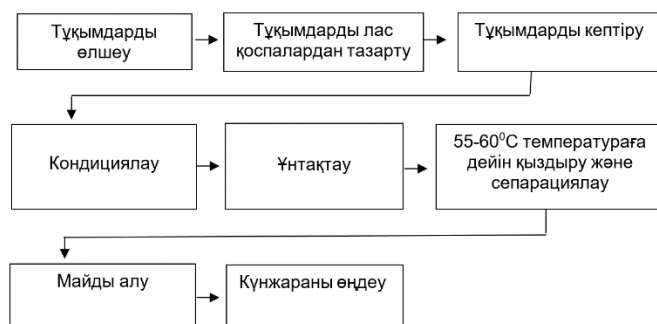
Сурет 1 – Қауын мен асқабақ тұқымдарынан май алудың технологиялық схемасы
