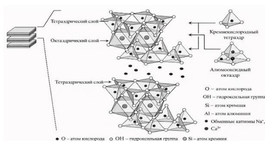
Рисунок 1 – Молекулярная (слоистая) структура монтмориллонита [16]
