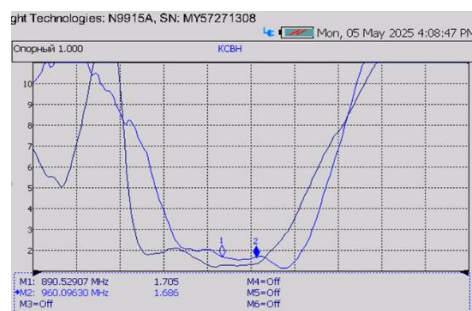
КСВ образца плоской антенны № 2
