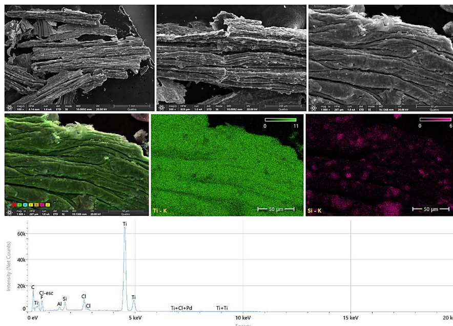
Рисунок 3 – СЭМ-изображение и ЭДС-спектр нанокompозита Ti_3C_2T_x с биогенным кремнием из рисовой шелухи
