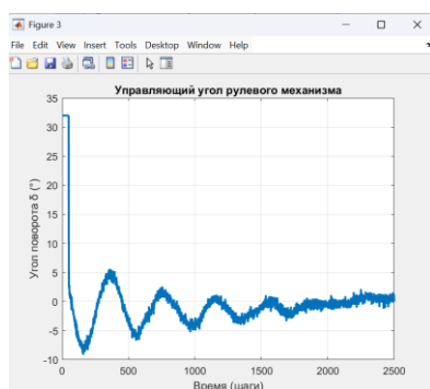
Рисунок 3 – Поведение управляющего угла \delta(t)
