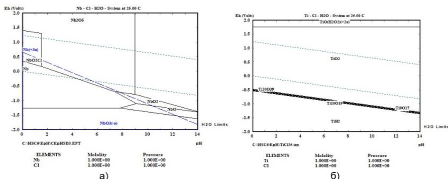
Рисунок 5 – диаграмма Пурбе систем Nb-Cl-H 2 O (а) и Ti-Cl-H 2 O (б)
