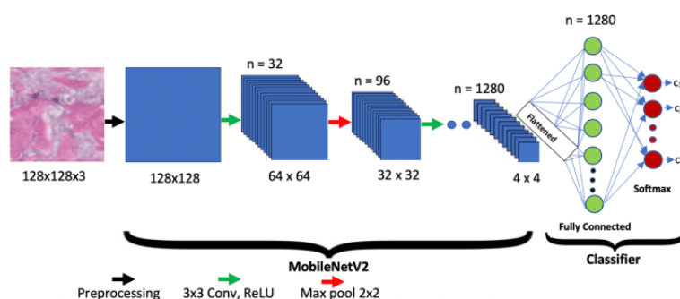
Сурет 2 – Мобильді желі архитектурасының визуалды көрінісі
