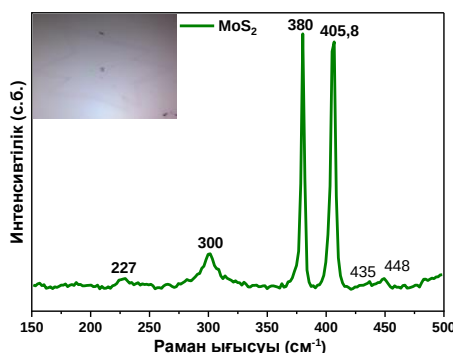
Сурет 7 – MoS 2 үлгісінің Раман спектрі
