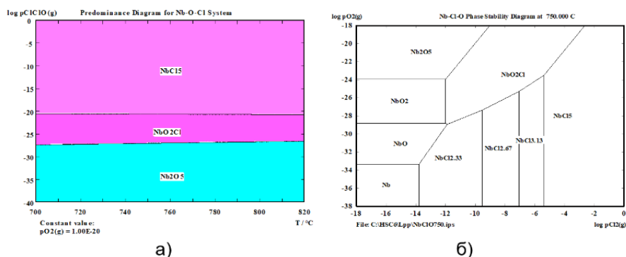
Рисунок 4 – Диаграмма T_{pp} в диапазоне температур 700-820 °C (а) и L_{pp} при температуре 750°C (б) системы Nb-Cl-O
