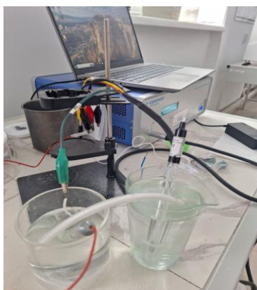
Рисунок 18 – Собранная электрохимическая установка
