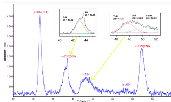
Рисунок 1 – GIXRD-дифрактограмма исходного многослойного покрытия (TiAlSiY)N/CrN при угле падения 15^\circ
