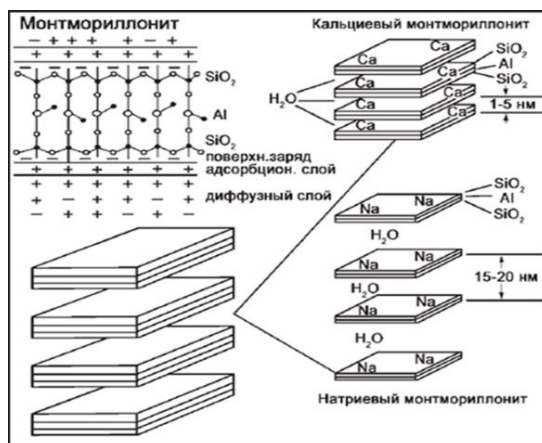
Рисунок 2 – Схема строения кальциевого и натриевого монтмориллонитов
