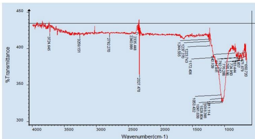
Рисунок 5 – ИК-спектр катализатора \text{Al}(2.5)\text{NaMM}+\text{HY}+\text{HZSM-5}
