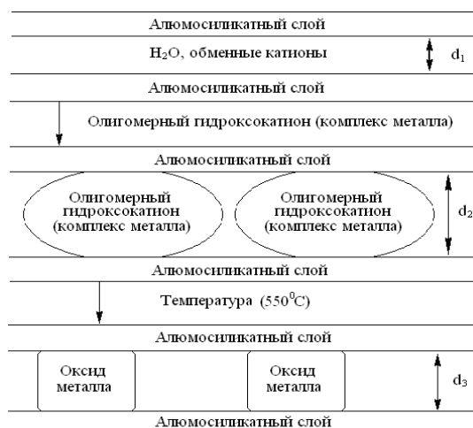
Рисунок 1 – Схематическое изображение процесса получения пилларированного слоистого алюмосиликата
