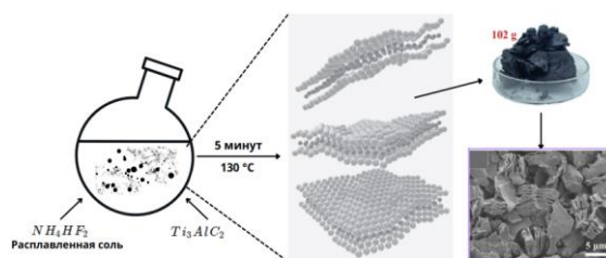
Рисунок 2 – Схема травления MXene с использованием расплавленной соли NH_4HF_2 .
