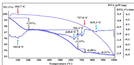
Сурет 1 – Зерттелетін цеолит үлгісін DTT / TG талдау (сәйкесінше DTT және DTG қисығындағы эндотермиялық шыңдары қызыл және көк бағдар сызықтарымен көрсетілген)
