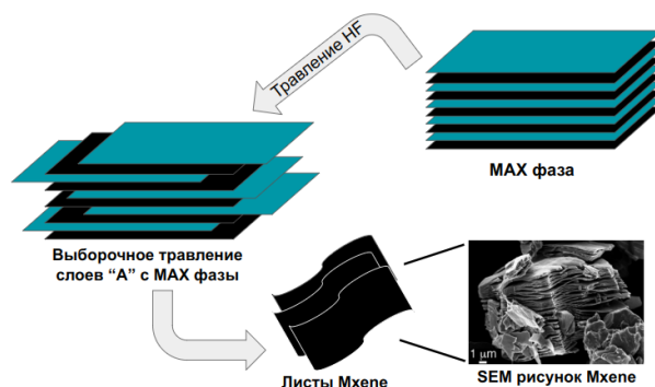
Рисунок 1 – Традиционный метод травления MAX фазы и получения листов Мхепе.
