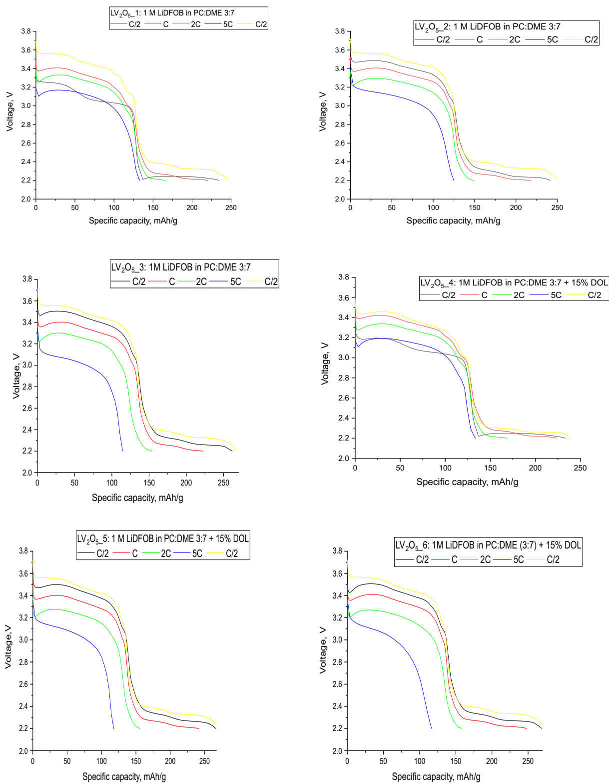
Сурет А.3 – Әртүрлі ток мәндеріндегі электрохимиялық ұяшықтардың разрядтық қисықтары, 1 бет
