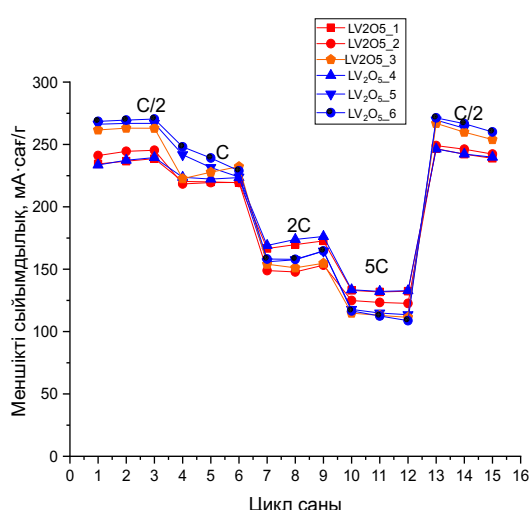
Сурет А.1 – Li-V 2 O 5 жүйесіндегі әртүрлі электролиттік құрамдар үшін электрохимиялық ұяшықтардың әртүрлі тоқтық режимдердегі (C/2, C, 2C және 5C) меншікті сыйымдылықтарының цикл санына тәуелділігі, 1 бет
