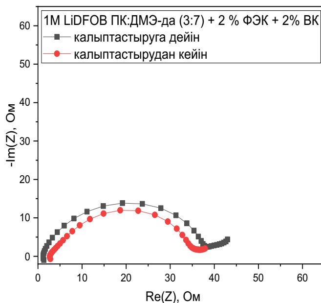
Сурет 19 - Ұяшықтардың қалыптастыру кезеңіне дейін және кейін түсірілген импеданстық диаграммасы
