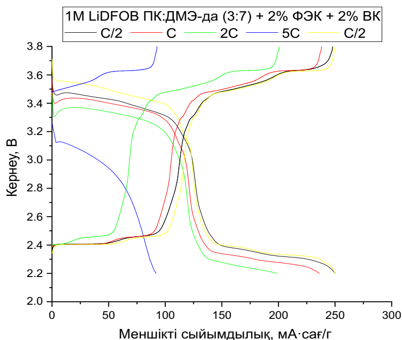
Сурет 15 – Тоқтың әртүрлі мәндеріндегі ұяшықтардың заряд-разряд қисықтары
