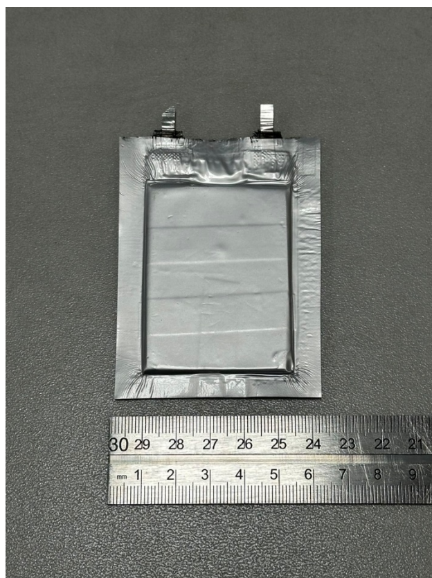
Сурет 33 – Жиналған элемент прототипінің фотосуреттері
