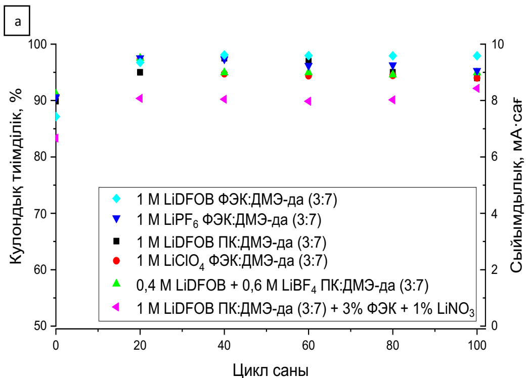
Сурет 29 – Әр түрлі температурада Cu-NMC 111 негізіндегі анодсыз ұяшықтардың Кулондық тиімділігі мен сыйымдылығы а) 30 °С; б) 60 °С,
