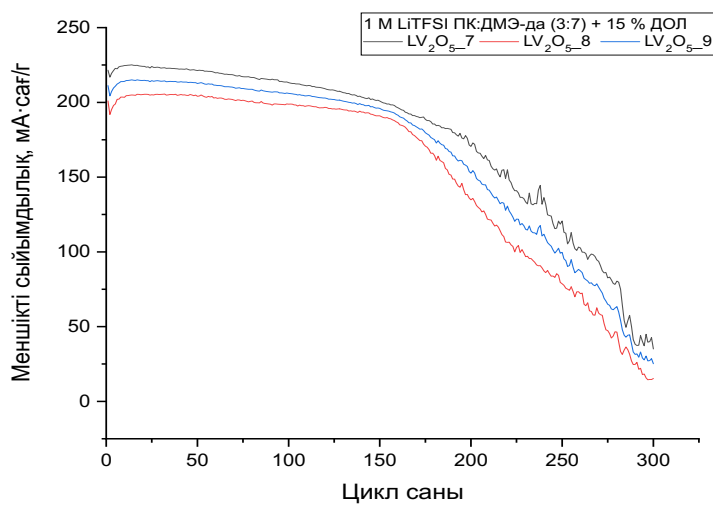
Сурет А.2 – Li-V 2 O 5 электрохимиялық жүйесінің үш бірдей ұяшығы үшін меншікті сыйымдылықтың цикл санына тәуелділігі
