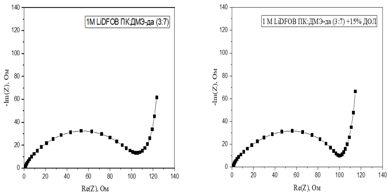
Сурет 31 – \text{Li-CF}_x негізіндегі біріншілік элементтердің импеданстық сипаттамалары, 1 бет
