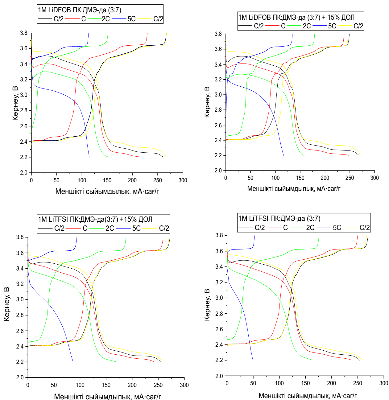
Сурет 12 – Тоқтың әртүрлі мәндеріндегі ұяшықтардың заряд-разряд қисықтары
