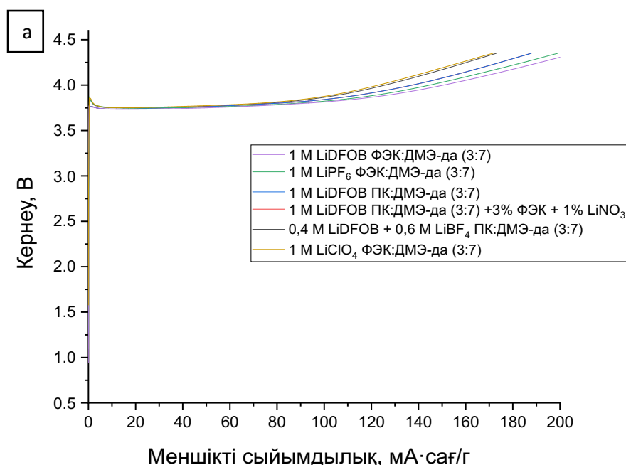
Сурет 27 – Өртүрлі электролиттері бар ұяшықтардың заряд қисықтары, температуралық режим: а) 30 °С; б) 60 °С, 1 бет
