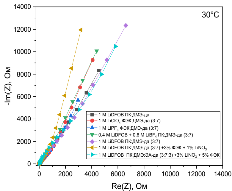
Сурет Г.1 – Әр түрлі температуралық режимдерде блоктаушы электродтары бар өлшеу ұяшығында алынған электролиттердің импеданстық диаграммалары, 1 бет
