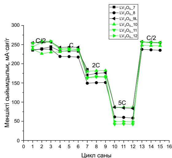
Сурет А.1 – Li-V 2 O 5 жүйесіндегі әртүрлі электролиттік құрамдар үшін электрохимиялық ұяшықтардың әртүрлі тоқтық режимдердегі (C/2, C, 2C және 5C) меншікті сыйымдылықтарының цикл санына тәуелділігі, 1 бет
