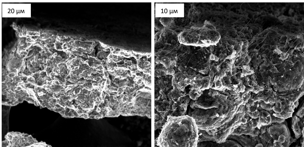
Сурет 30 – CF x негізіндегі катод бетінің СЭМ суреттері: 20 мкм масштабта; 10 мкм масштабтағы құрылымның үлкейтілген фрагменті
