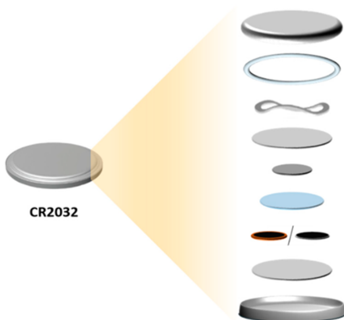
Сурет 7 – CR2032 форматындағы дискілік қуат элементінің және оның құрамдас бөліктерінің сызбалық бейнесі
