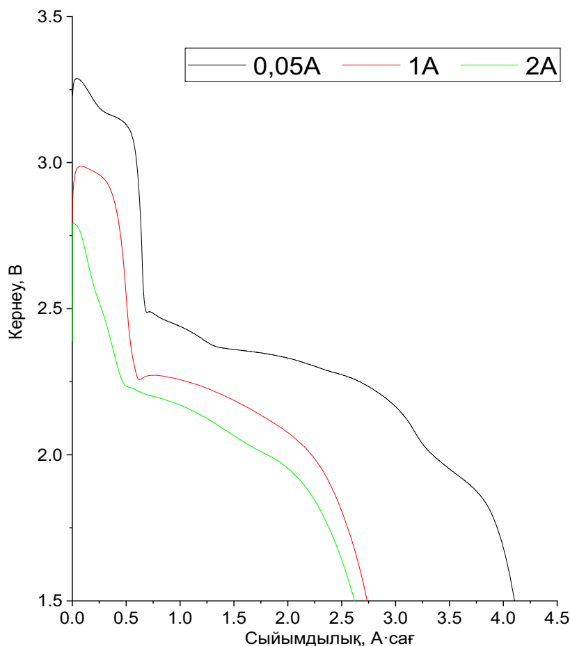
Сурет 34 – Өртүрлі тоқтық режимдерде Li–V 2 O 5 /CF x негізіндегі литийлік тоқ көзі прототипінің разрядтық сипаттамалары
