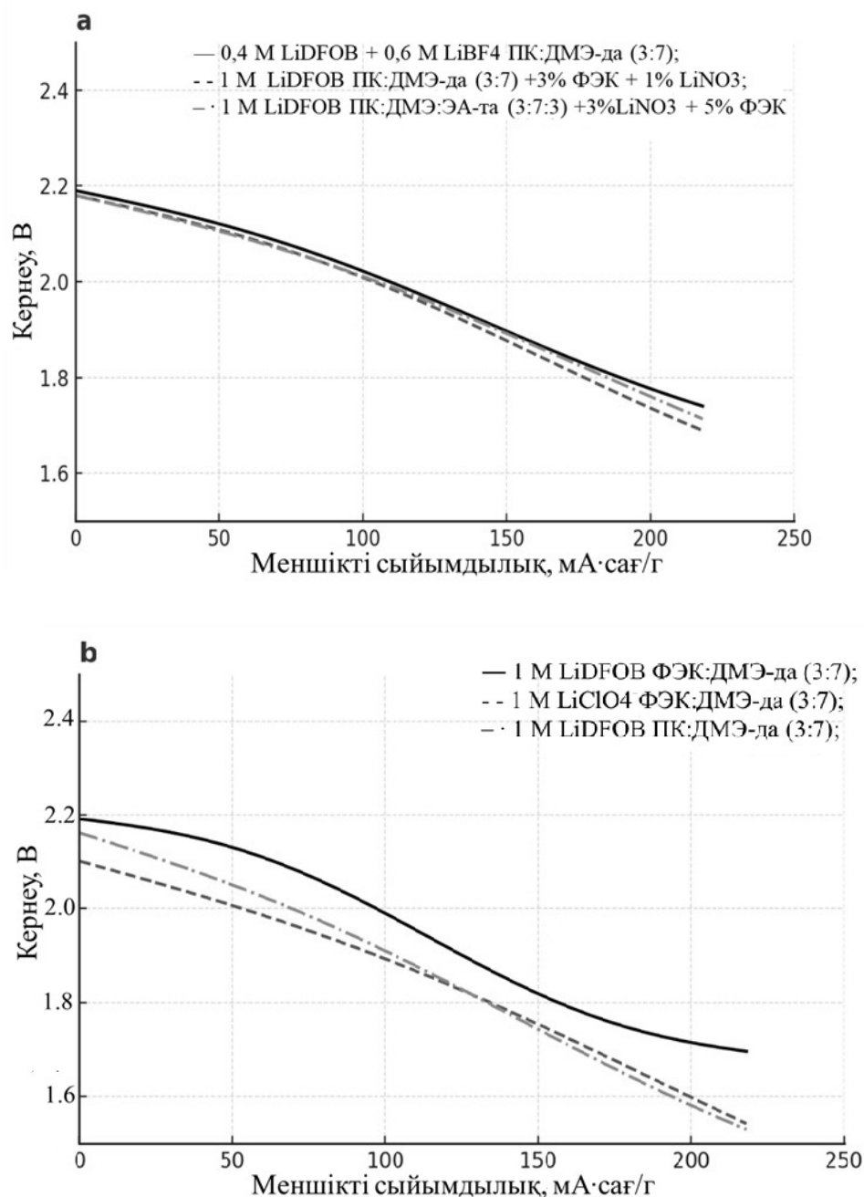
Сурет 32 – -20\text{ }^{\circ}\text{C} \text{Li-CFx} негізіндегі ұяшықтардың разрядтық қисықтары
