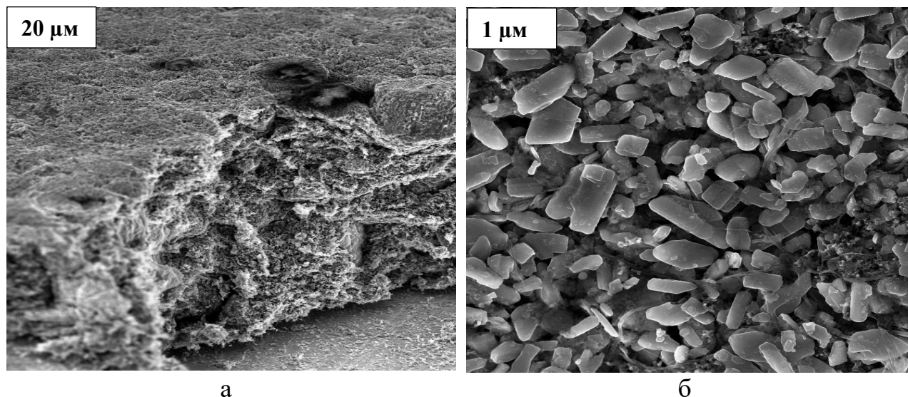
а) - жабынның біркелкі таралуын көрсететін беттің жалпы көрінісі; (б) - микрокеуекті құрылымы бар үлкейтілген аймақ
