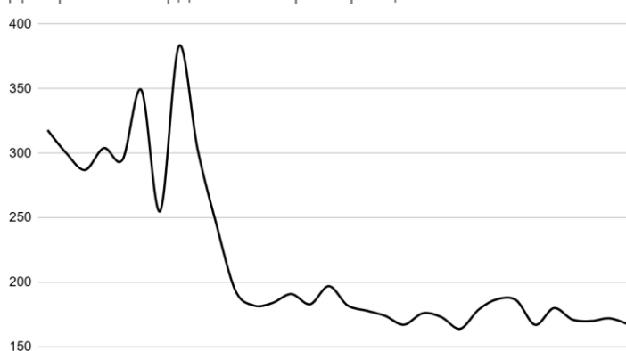
Диаграмма твердости шлифа образца стали 20ГЛ №2
